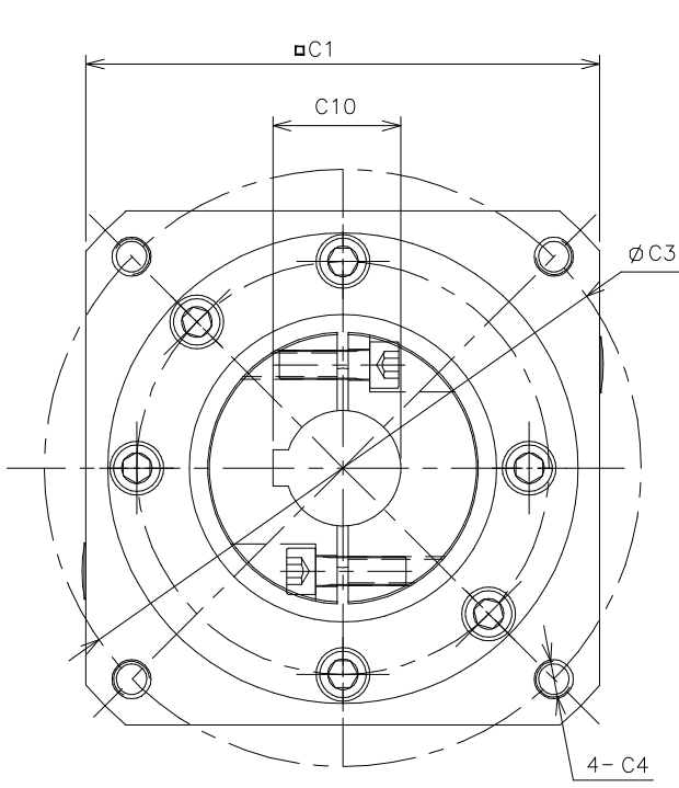
输入端
