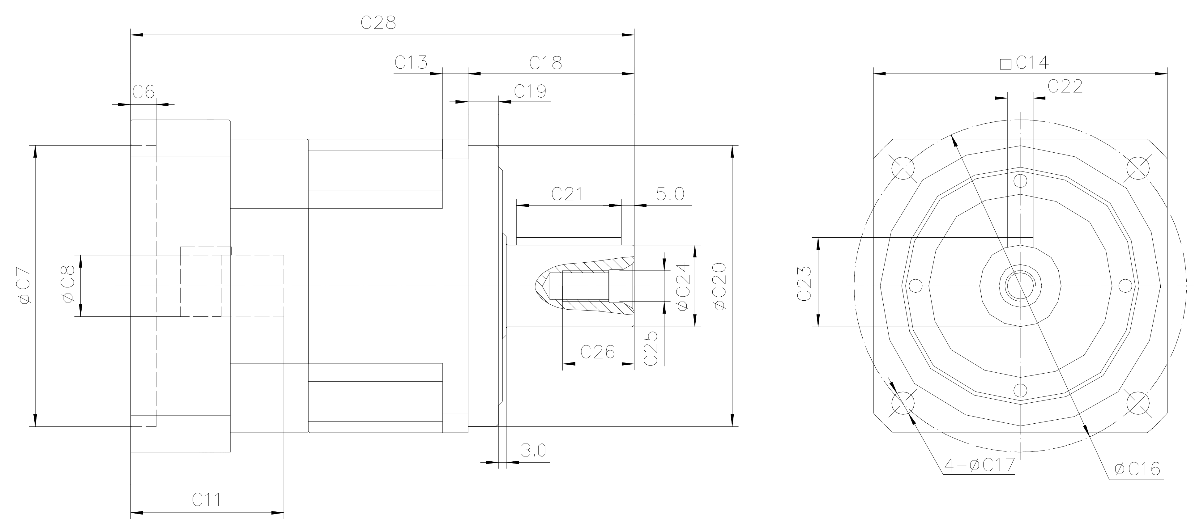
输出端
