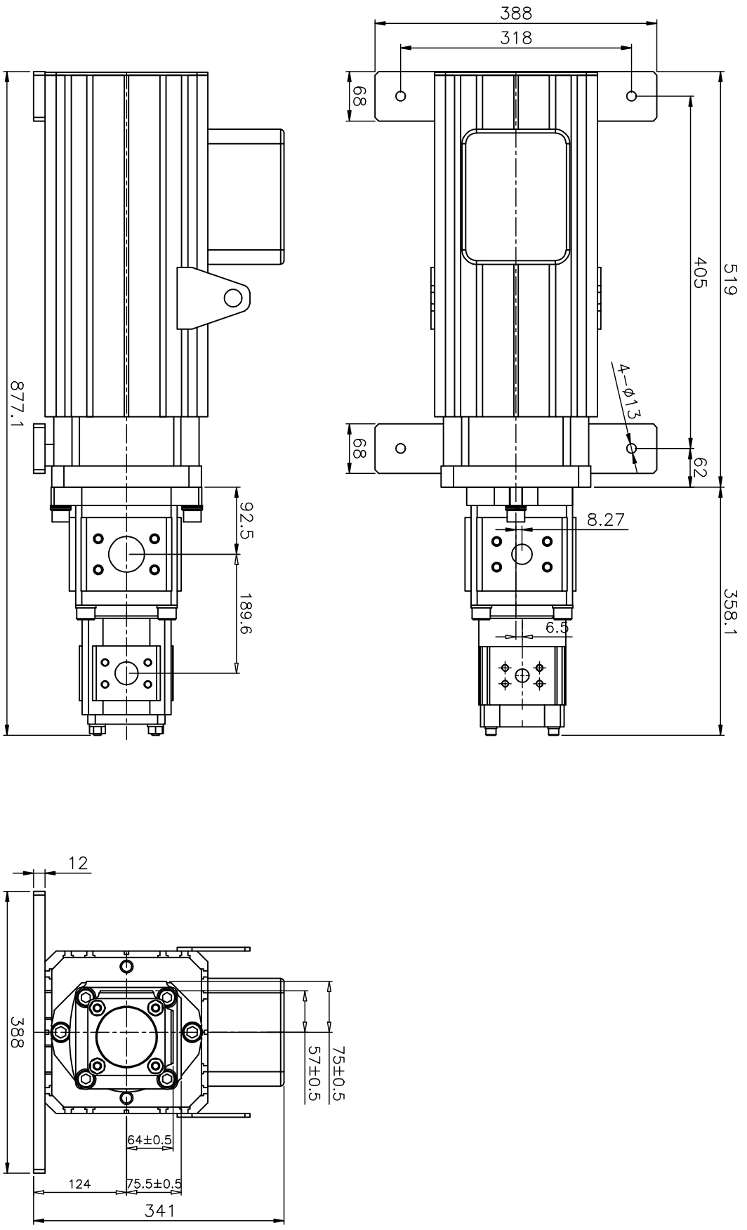
80+40cc+U1010F 安装尺寸图
