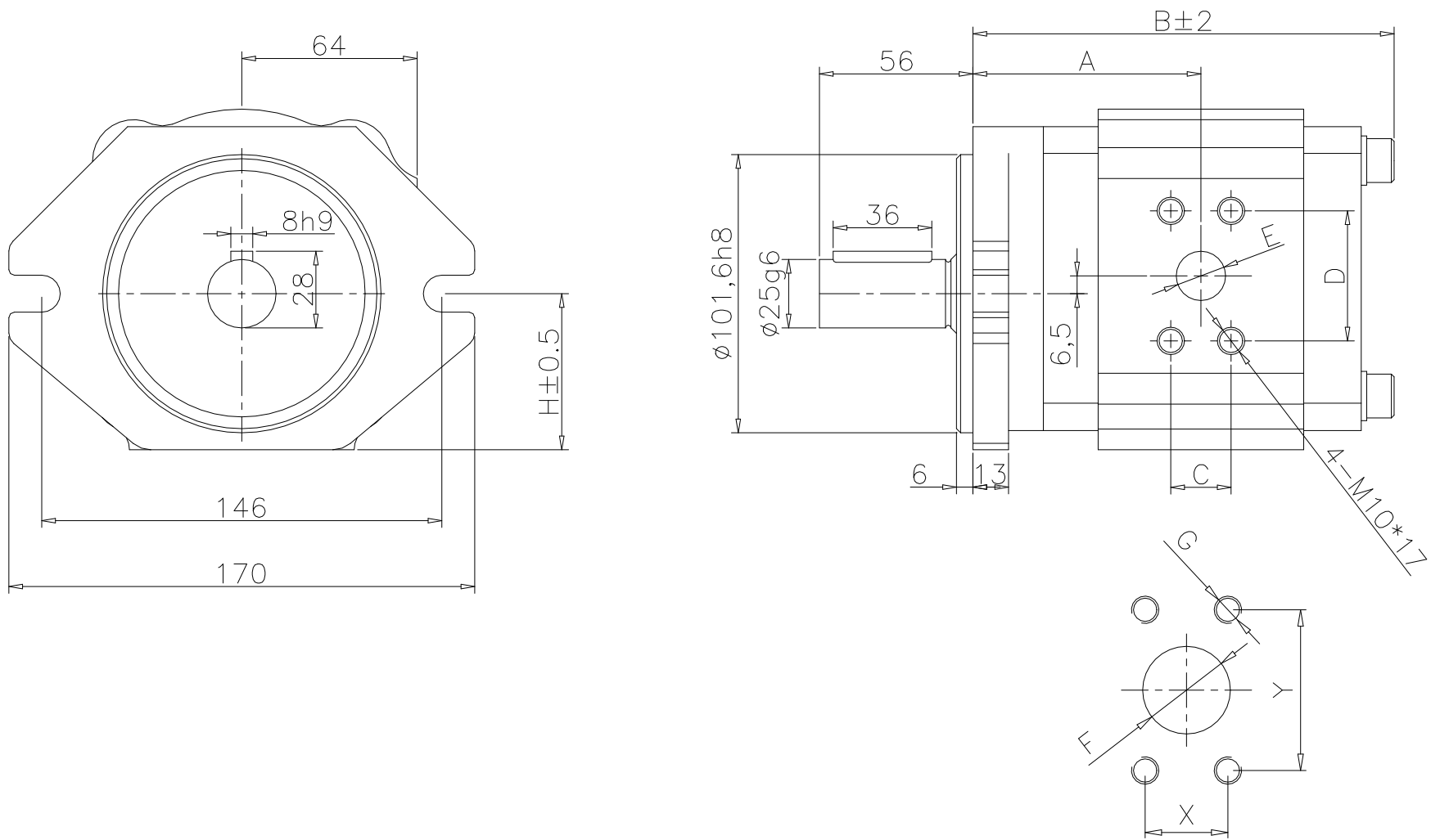
EIPC3平键泵安装尺寸图
