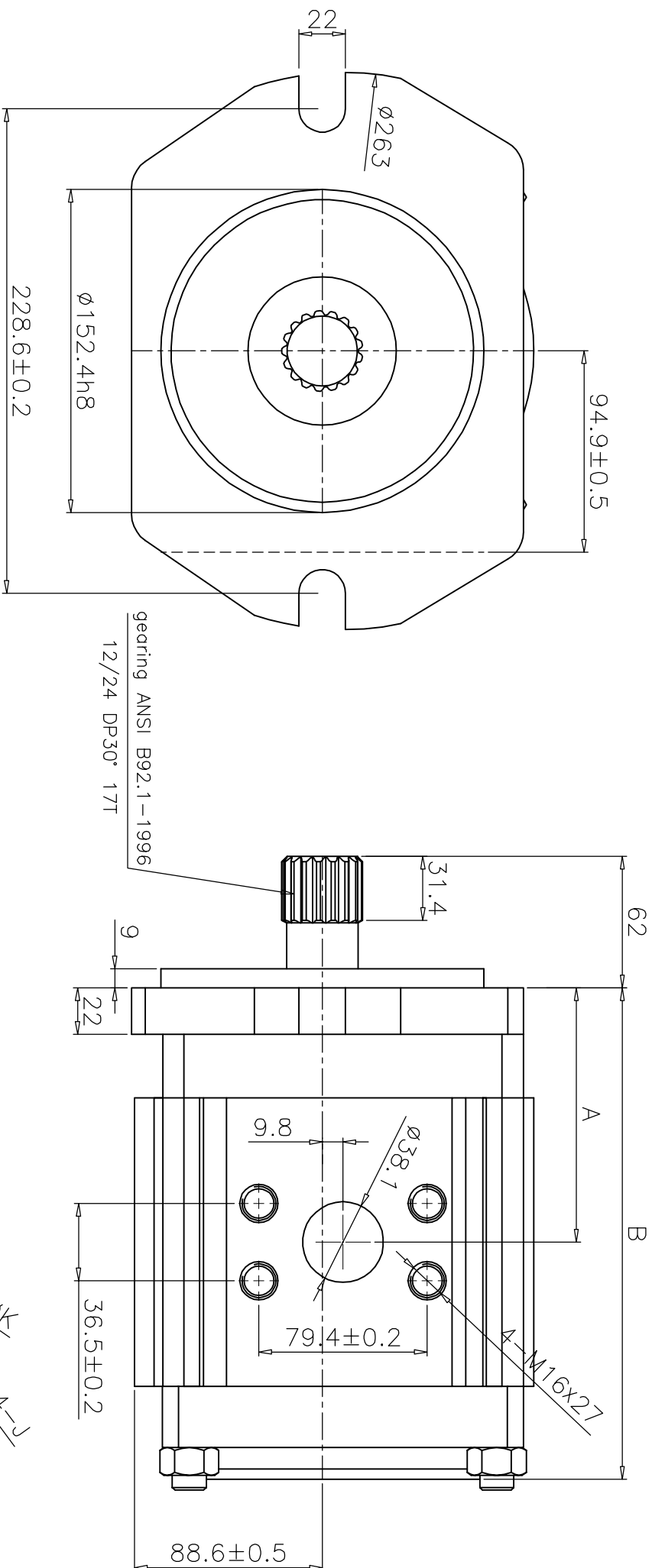
EIPC6花键油泵外形及安装尺寸图
