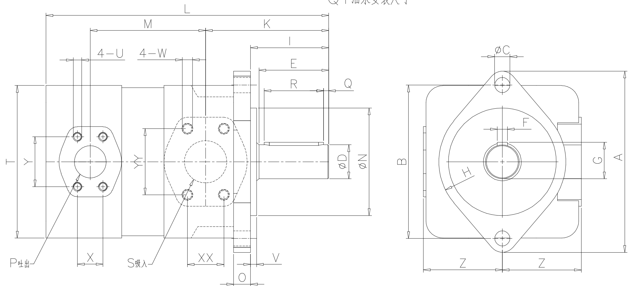
QT油泵安装尺寸
