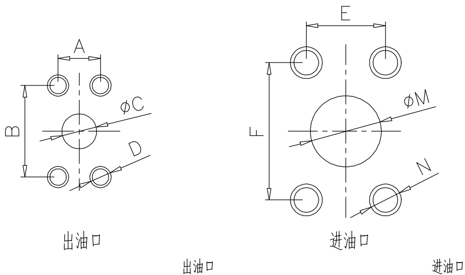
油泵进出油口法兰尺寸图
