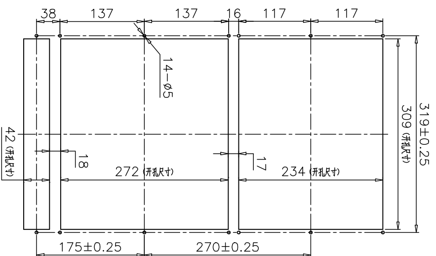
TMP3360 安装尺寸图
