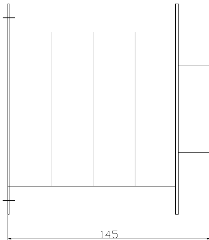
350W、660W 隔离变压器安装孔位尺寸图
