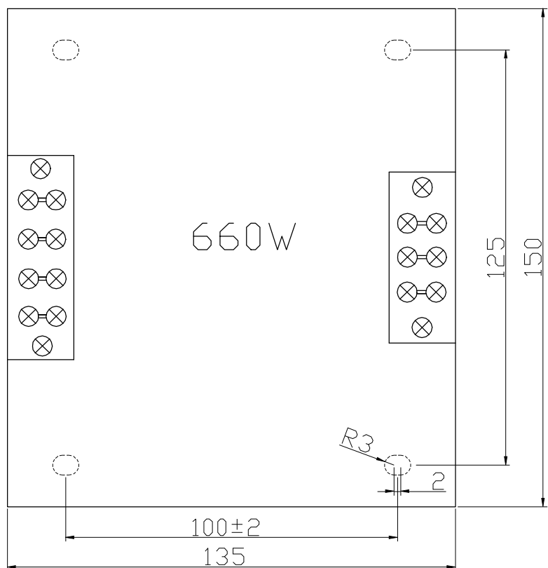
350W、660W 隔离变压器安装孔位尺寸图
