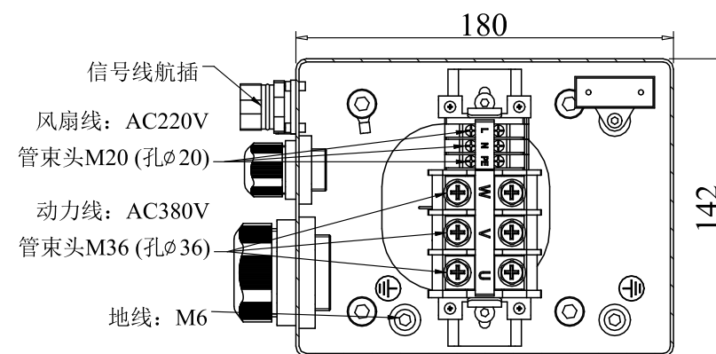
A-A接线盒
