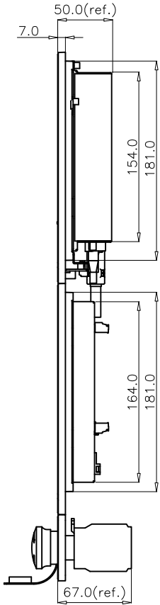
TMA26481 鋁材面板 外觀尺寸圖
