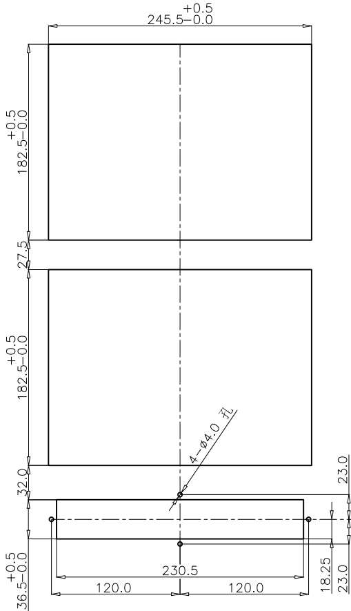
TMA26481 鋁材面板 安裝尺寸圖
