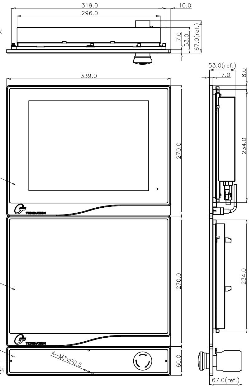
TMA33601 鋁殼面板外觀尺寸圖
