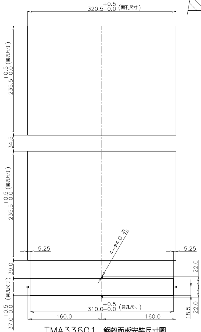
TMA33601 鋁殼面板安裝尺寸圖
