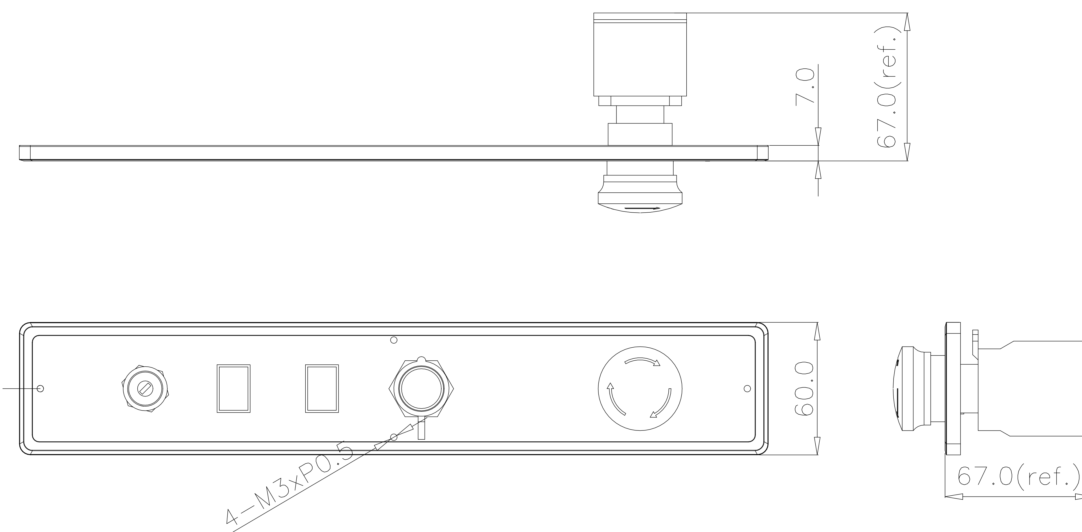
TMA33601 鋁殼面板急停區外觀尺寸圖
