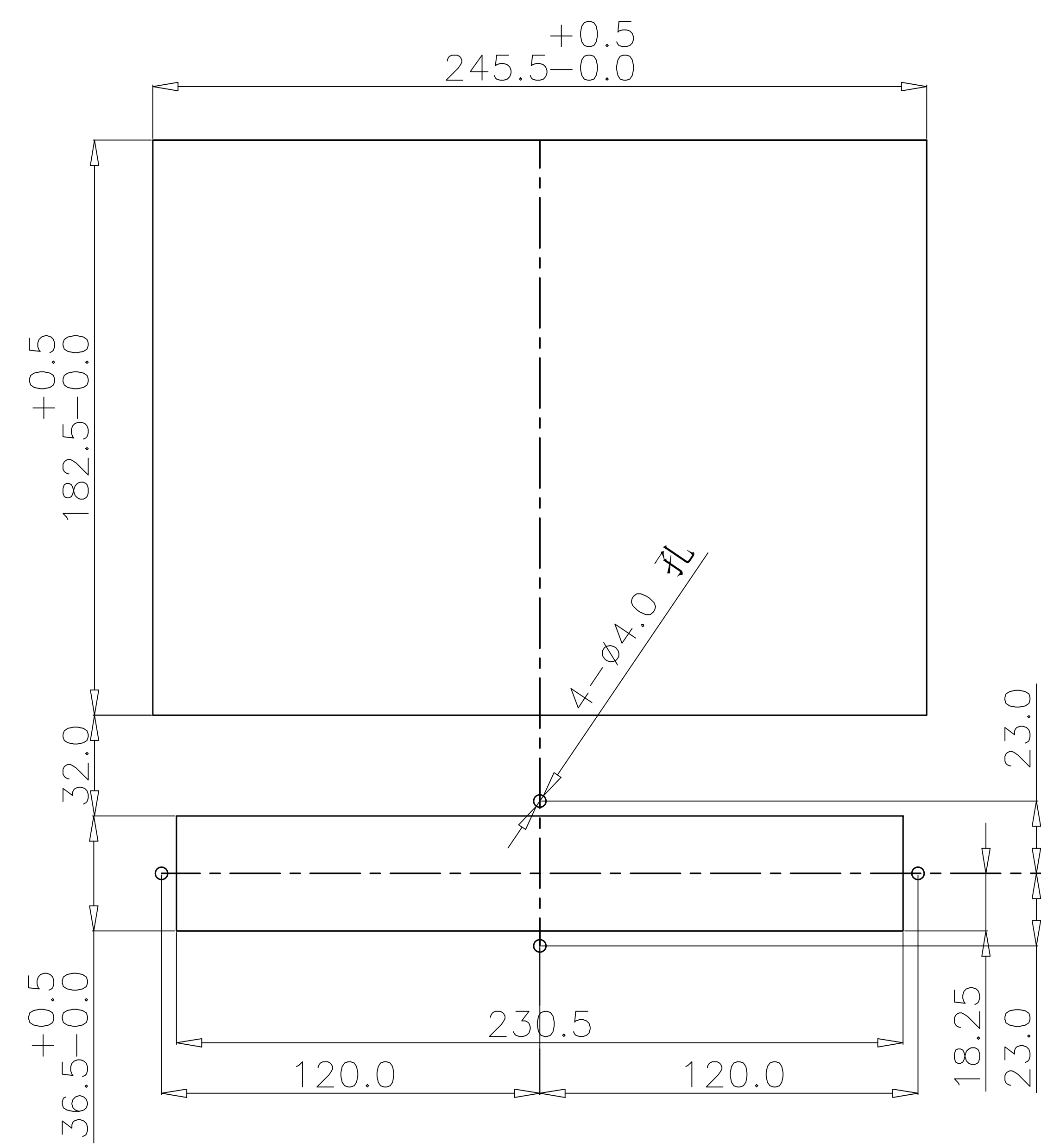
鋁殼Q8(TOUCH) 安裝尺寸圖
